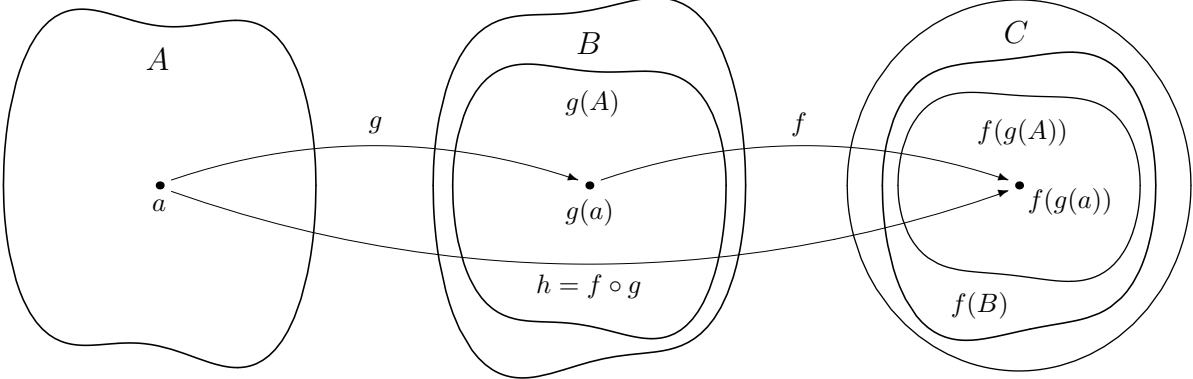
Abb. 5.1 Verkettung von f und g
