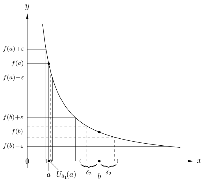
Abb. 6.14 Für das gleiche \varepsilon > 0 kann hier kein universelles \delta > 0 gewählt werden. Je näher man sich mit a dem Wert 0 nähert, desto kleiner muß die entsprechende \delta -Umgebung genommen werden, damit die \delta -Umgebung von a in die \varepsilon -Umgebung von f(a) abgebildet wird. \delta hängt sowohl von a als auch von \varepsilon ab.
