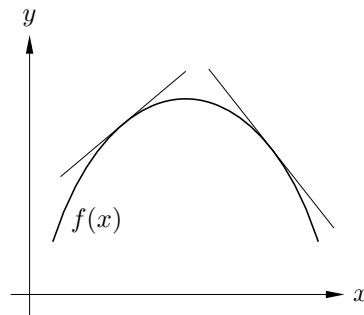
Abb. 7.10 b f(x) ist streng konvex von oben
